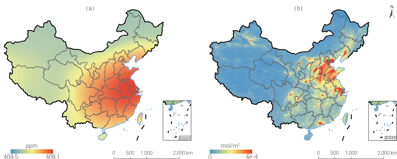
图 5-3. (a) 2018 年 \text{CO}_2 平均浓度；(b) 2019 年 \text{NO}_2 年度平均浓度
