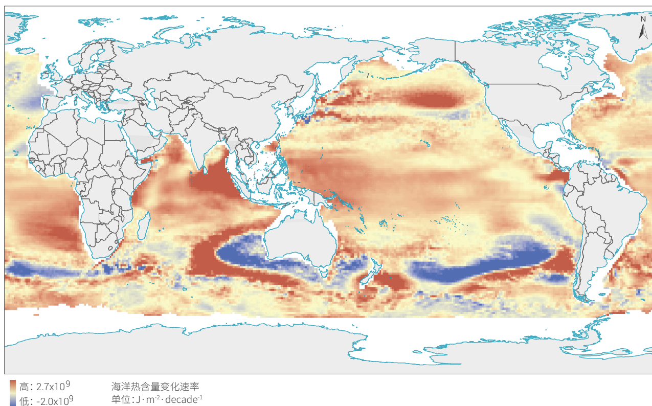
图 5-10. 1993~2020 年全球海洋上层 2000 m 热含量变化速率
